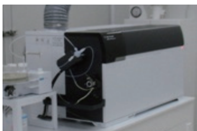
用于检测 wafer 表面金属污染
