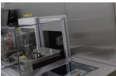
用于检测 wafer 厚度、平坦度等几何参数
